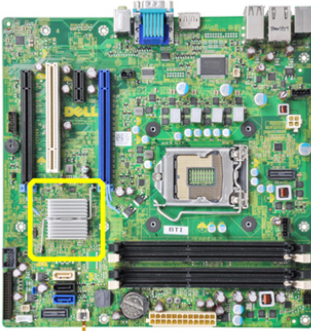
Slika 1. Ranija verzija matične ploče sa rashladnim elementom
